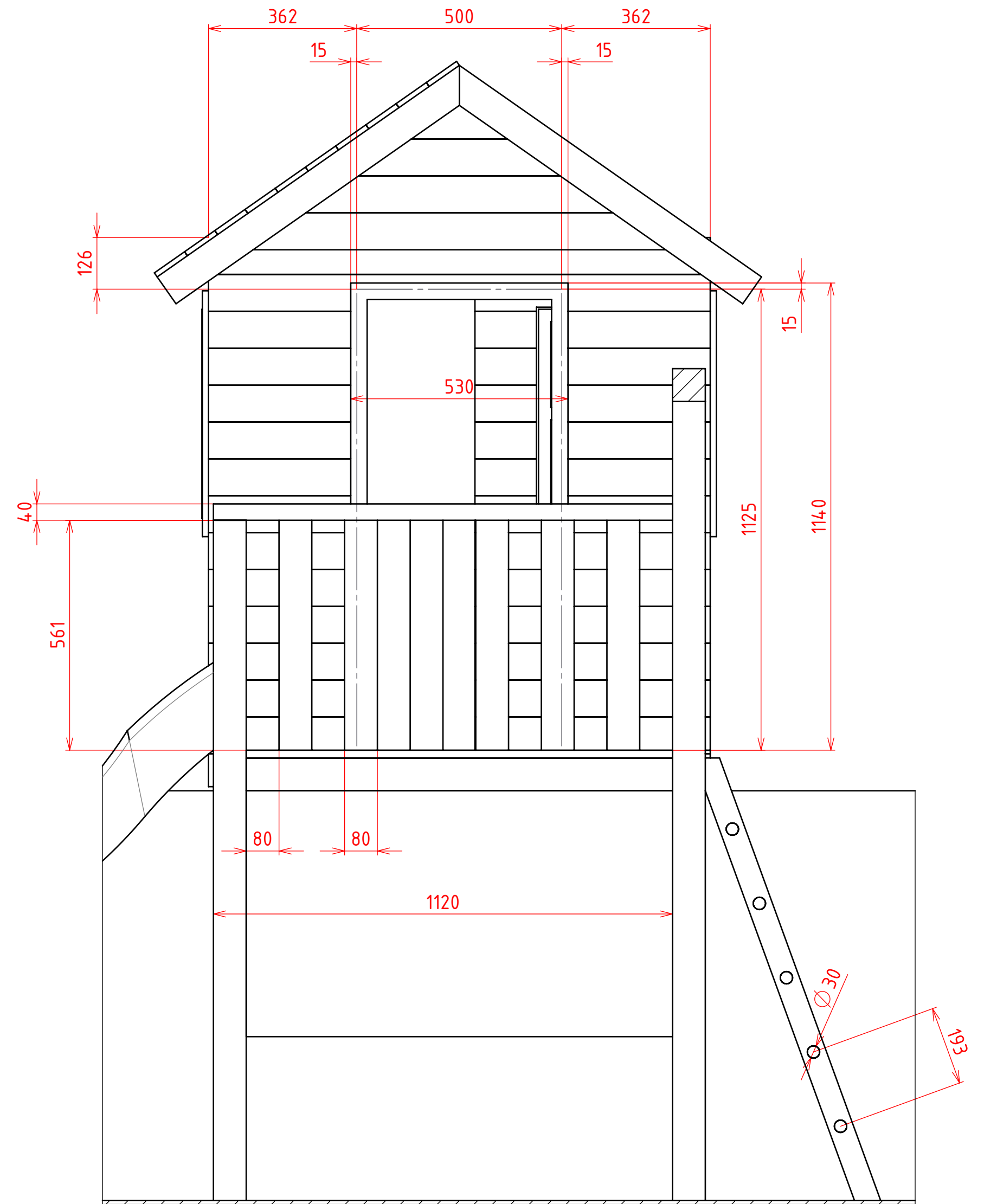
ŘEZ B-B
