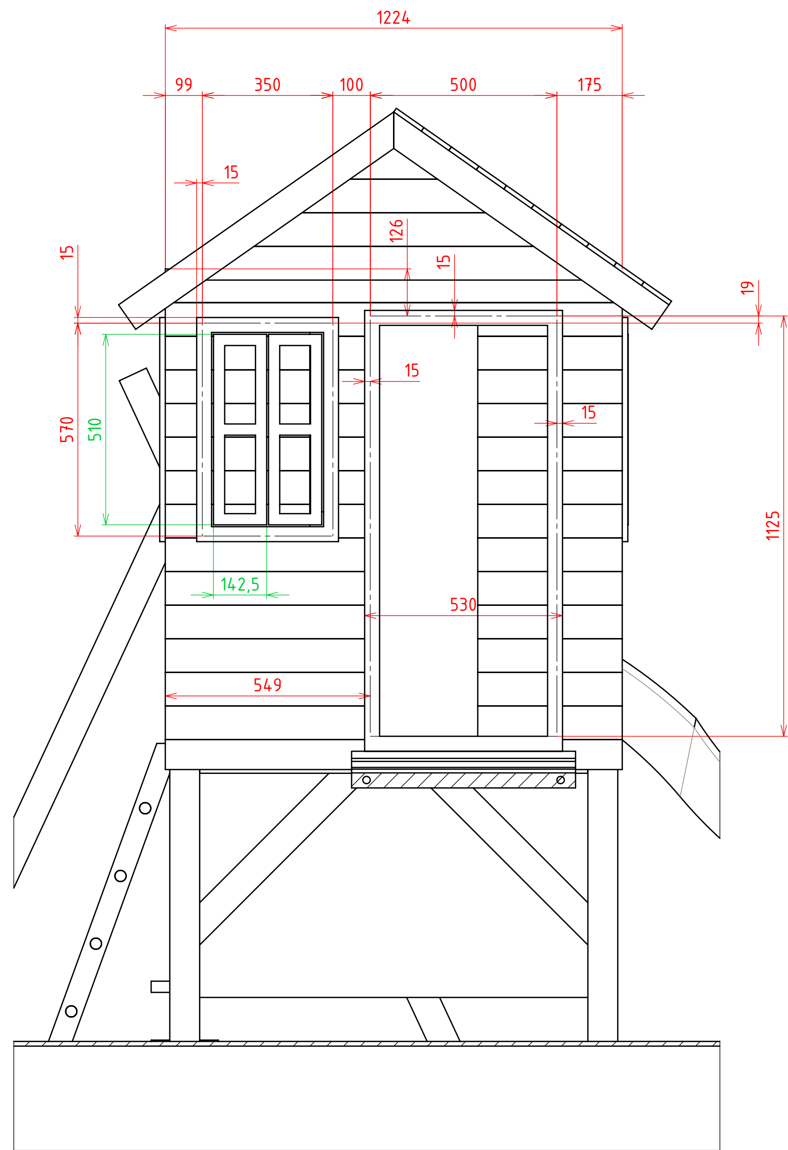
ŘEZ A-A
